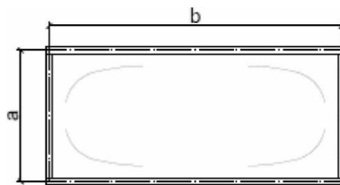
Рисунок В.1 - Схемы приложения нагрузки для испытания светопрозрачных покрытий и фонарей
